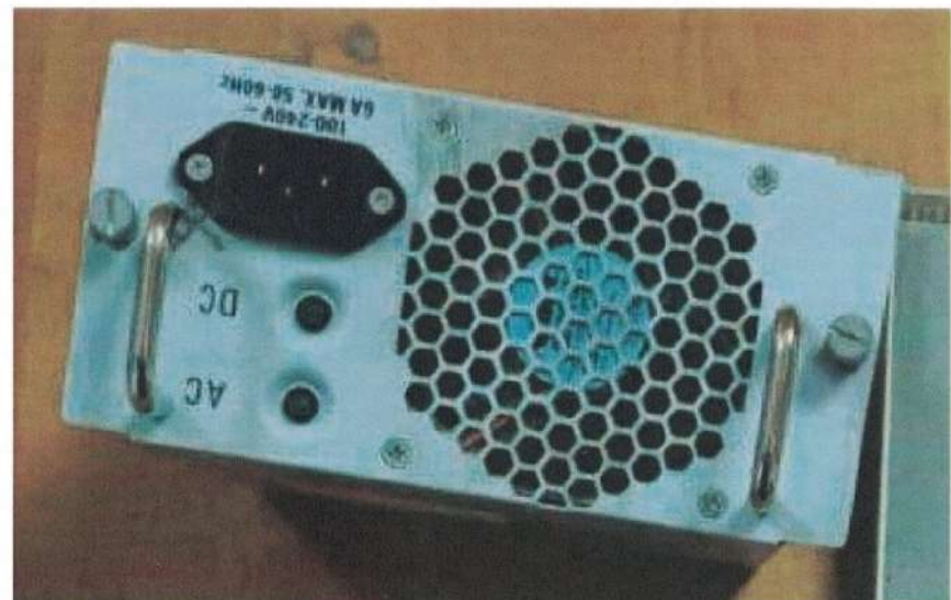
Рис. 3 - Резервне джерело живлення
