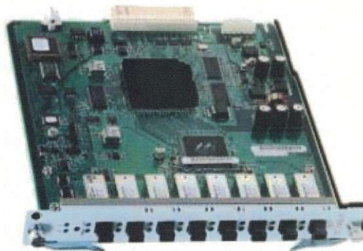
Рис. 7 - Модуль 3COM 3C16829 ETHERNET 100MBPS 8-PORTS
