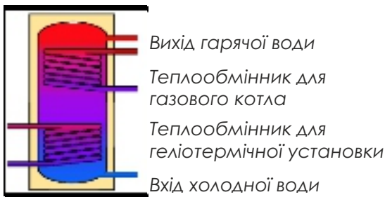
Рис. 184 Бівалентний бойлер непрямого нагріву
