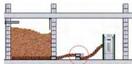
Рис.89 Схема збільшення довжини лінії паливоподачі за допомогою передавального пункту
