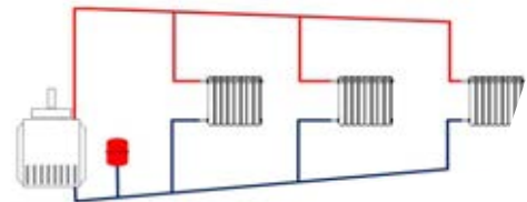
Рис.111 Система опалення з природною циркуляцією
