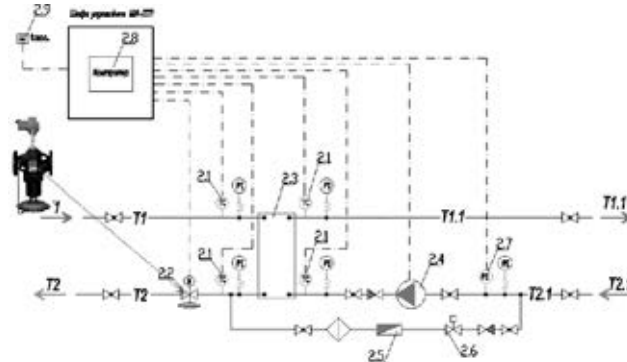
Рис. 147 «Незалежна» схема підключення до теплової мережі
