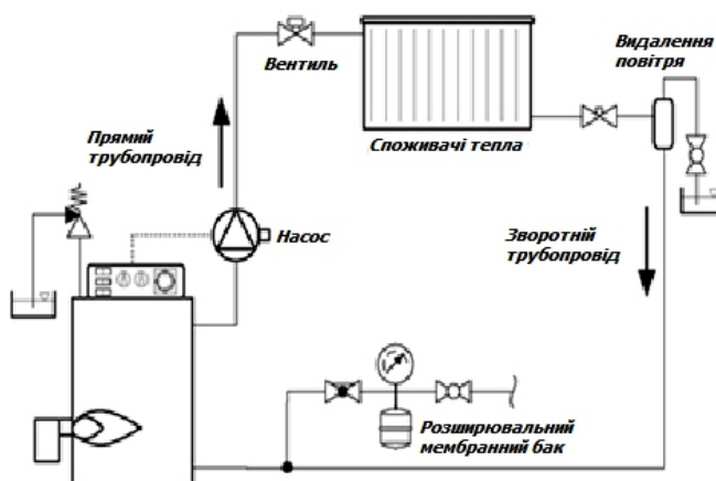
Рис.97 Гідралічна схема підключення насосу
