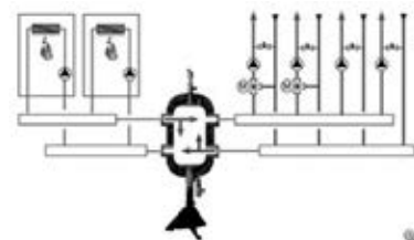
Рис.104 Гідрострілка
