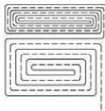
Рис.128 Метод укладання равилик з послідовно приєднаним контуром робочої зони
