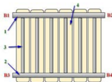
Рис. 28 Спрощена будова радіатора
