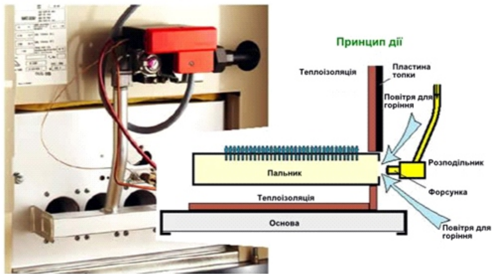
Рис.95 Атмосферний пальник
