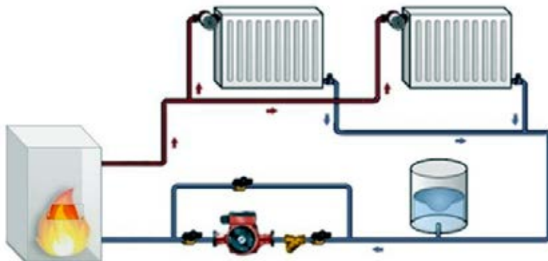
Рис.112 Система опалення з примусовою циркуляцією
