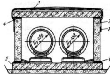
Рис. 139 Непрохідний канал із збірних залізобетонних плит і стінових блоків: 1 – плита перекриття; 2 – стіновий блок; 3 – гідроізоляція; 4 – цементний розчин; 5 – плита днища
