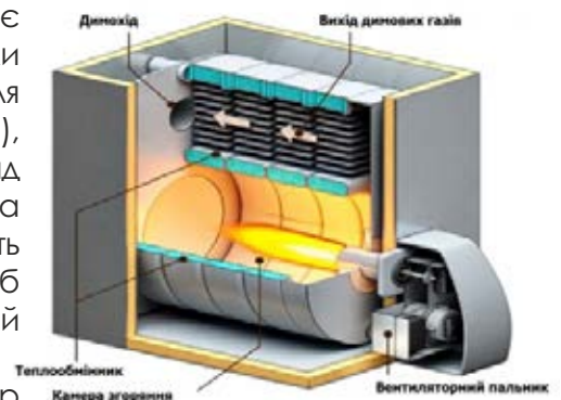
Рис.94 Рідкопаливний котел
