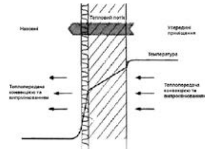
Рис.8 Теплопередача
