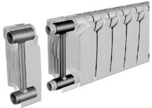
Рис.20 Біметалевий радіатор
