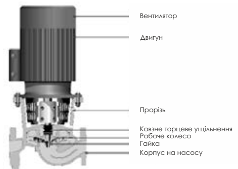
Рис.101 Конструкція in-line насоса с сухим ротором
