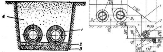
Рис. 140 Прокладання безканалних трубопроводів в глинистих ґрунтах: 1 – дренажна труба; 2 – пісок для дренажу; 3 – щебінь; 4 – пісок засипки; 5 – робочий дренаж із щебню; 6 – гідроізоляція
