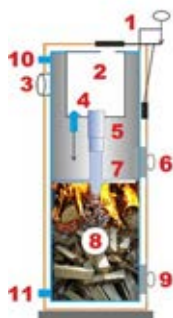
Рис.81 Котел тривалого горіння
