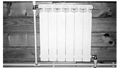
Рис. 156 Під'єднання радіатора
