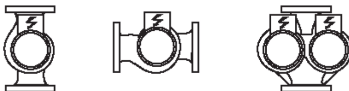
Рис.99 Припустимі способи установки без обмежень для насосів з безступінчастим регулюванням частоти обертання
