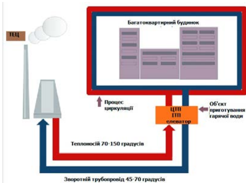
Рис.141 Схема теплопостачання
