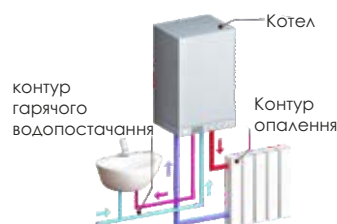
Рис.52 Двоконтурний котел
