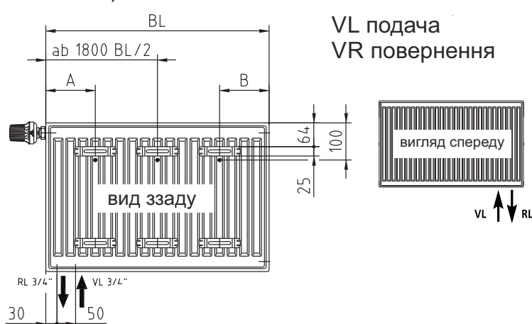
Рис. 11 Типи панельних сталевих радіаторів
