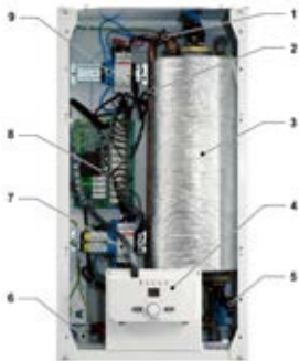
Рис.75 Будова електричного котла
