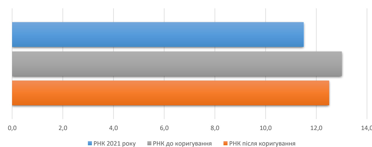
Коригування РНК
