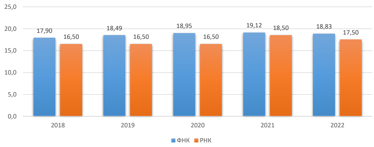
Коригування РНК
