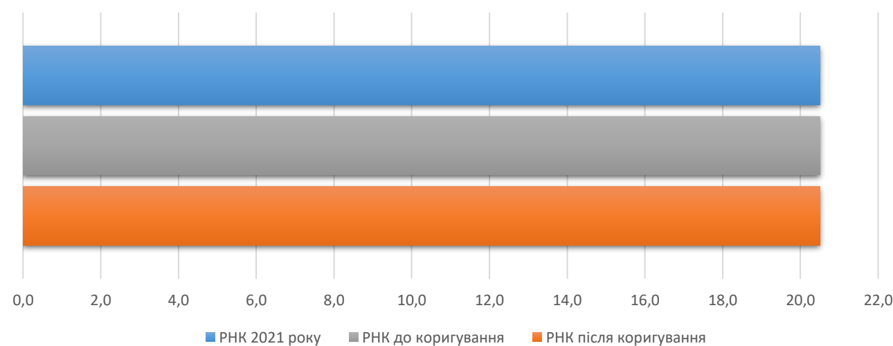
Коригування РНК
