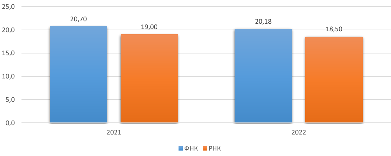
Коригування РНК
