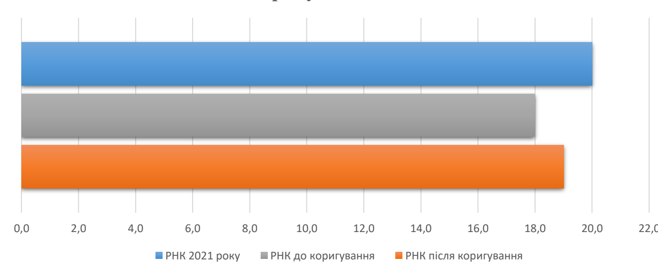
Коригування РНК
