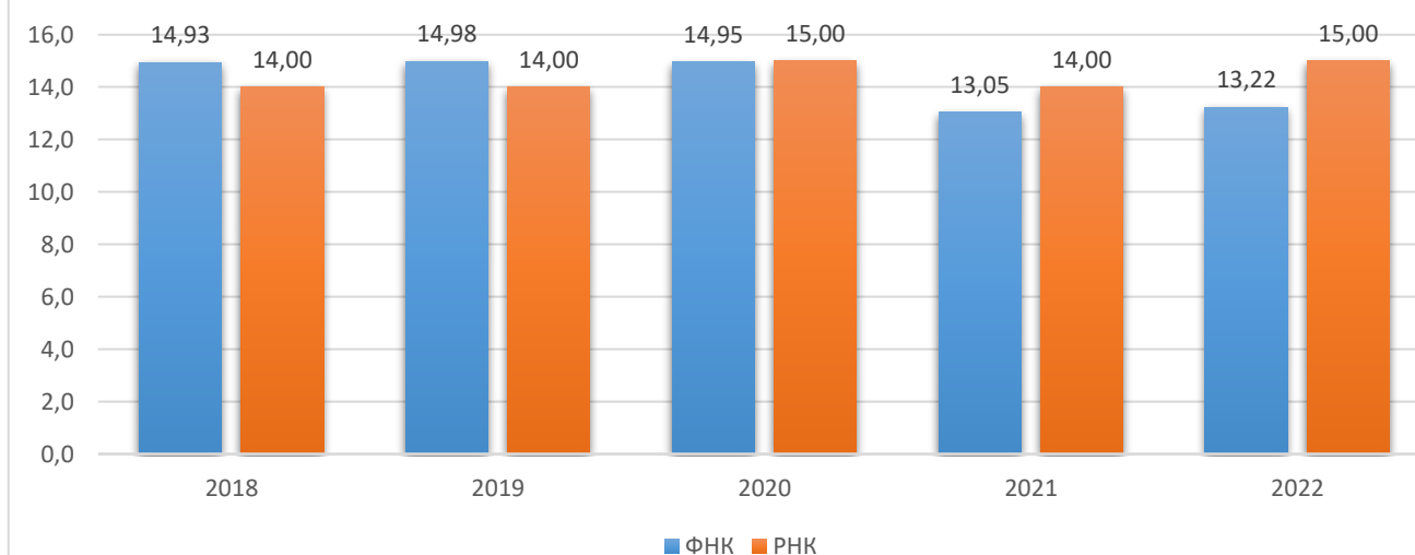
Порівняння ФНК з РНК
