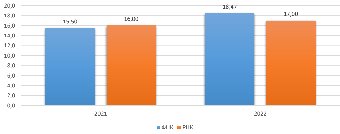
Коригування РНК
