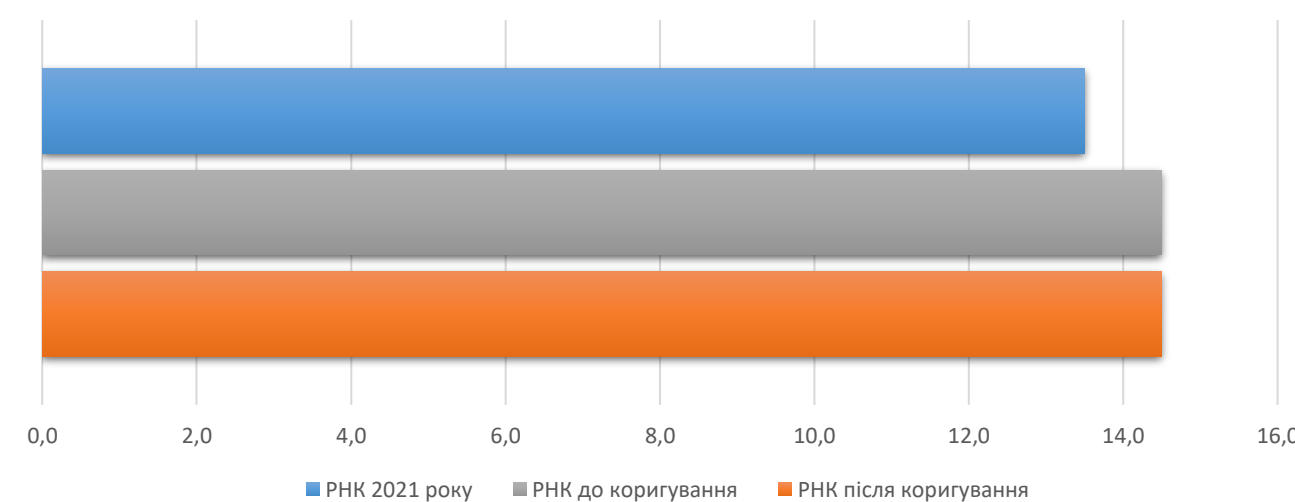
Коригування РНК
