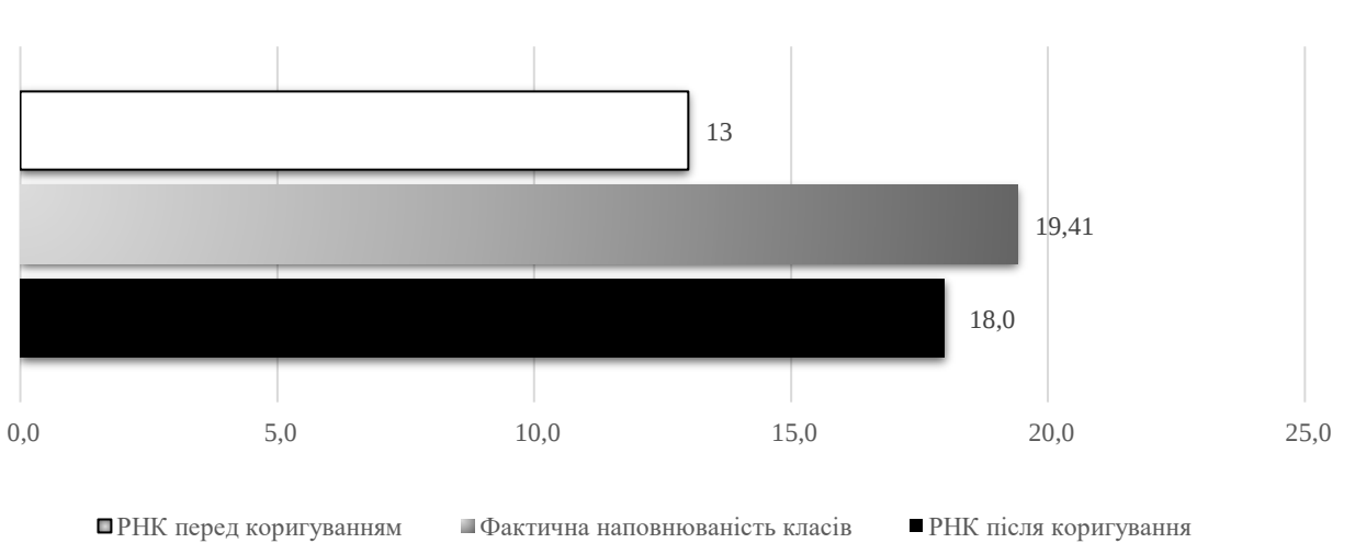
Коригування РНК
