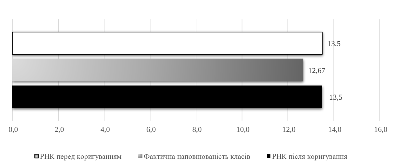
Коригування РНК
