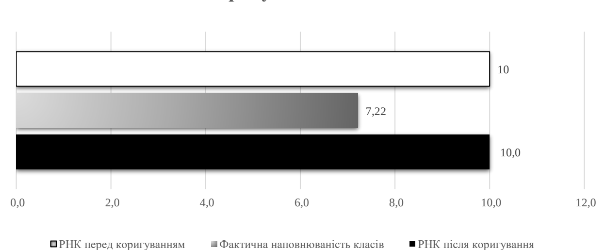
Коригування РНК
