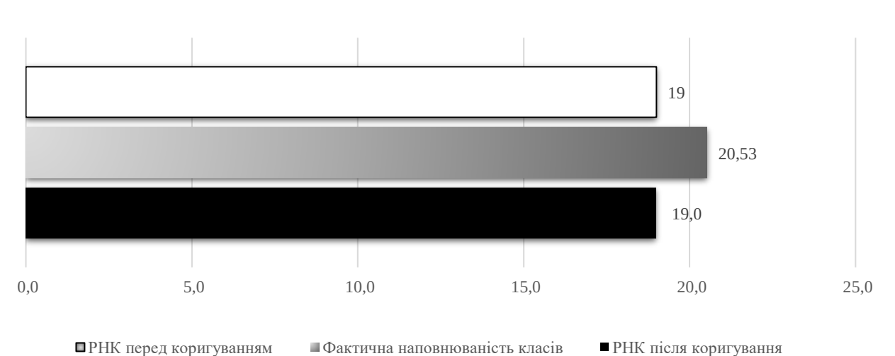
Коригування РНК
