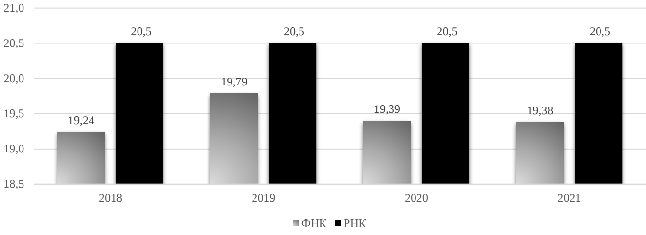
Коригування РНК
